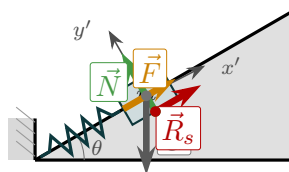
Figur 4.8: Kloss på skråplan ( \theta = 30 ) holdt av fjær \vec{F} og friksjon \vec{R}_s . Koordinatsystem: x' opp langs planet, y' normalt ut.
