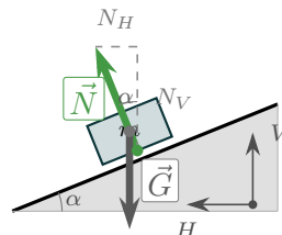
Figur 4.12: Dosert veibane i tverrsnitt. \vec{N} dekomponeres i N_V (opp) og N_H (inn mot sentrum). H -aksen peker inn mot svingssentrummet.
