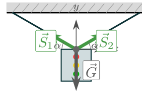
Figur 4.9: Trafikklys i ro. Snorkreftene \vec{S}_1 og \vec{S}_2 danner vinkel \alpha med horisontal.
