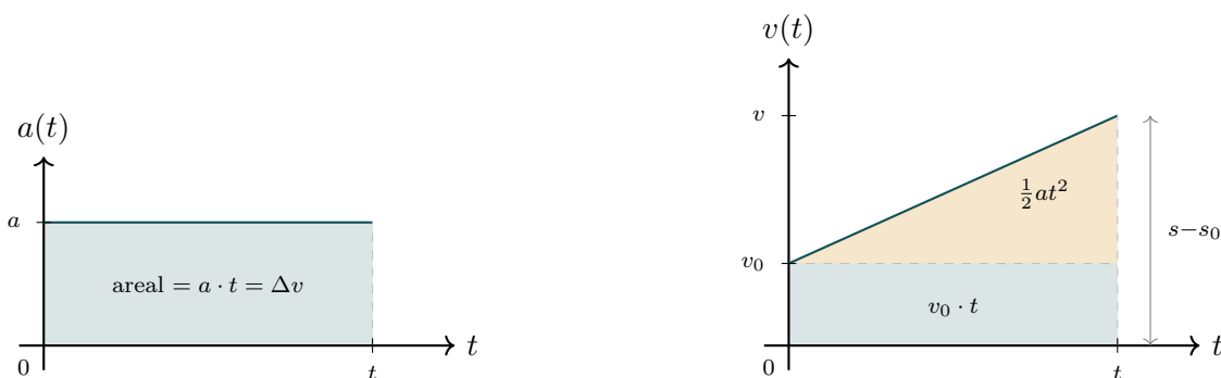
(a) a(t) -grafene. Arealet av rektangelet er endringen i fart: \Delta v = v - v_0 .
