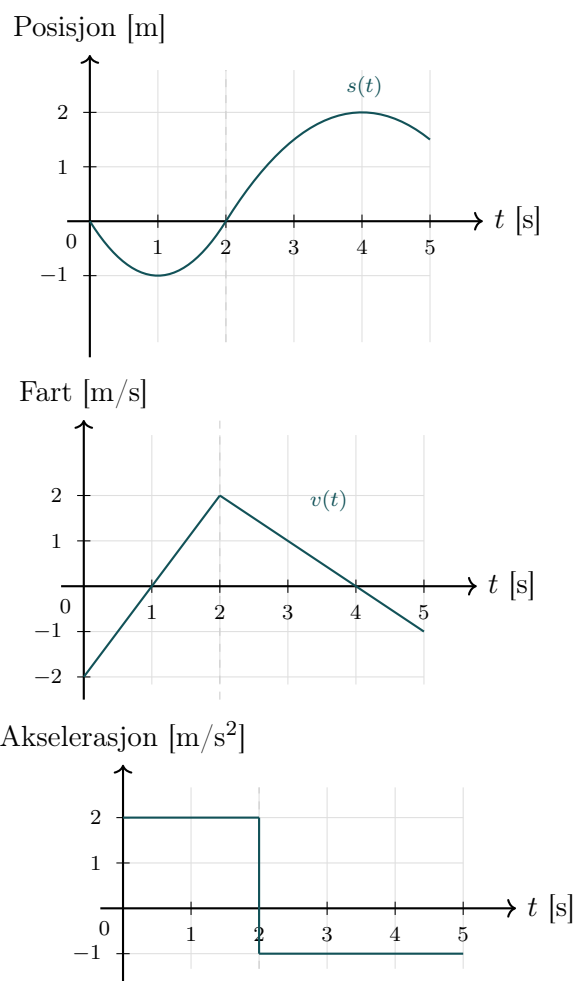
Figur 3.6: Posisjon, fart og akselerasjon ved varierende akselerasjon ( s_0 = 0 , v_0 = -2 \text{ m/s} ; a_1 = 2 \text{ m/s}^2 for t \in [0, 2 \text{ s}] og a_2 = -1 \text{ m/s}^2 for t \in [2, 5 \text{ s}] ).
