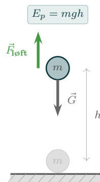
Figur 5.5: Masse m løftes mot tyngdekraften til høyde h . Arbeidet W = mgh lagres som potensiell energi.
