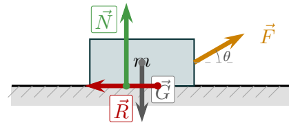
Figur 4.5: Kjelke dradd med kraft \vec{F} i vinkel \theta = 30 over horisontal. Friksjonskraften \vec{R} og normalkraften \vec{N} angriper ved kontaktflaten.
