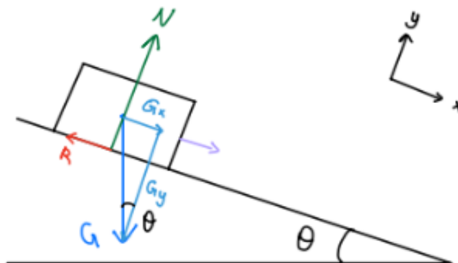
Figur 4.10: Krefter i skråplan
